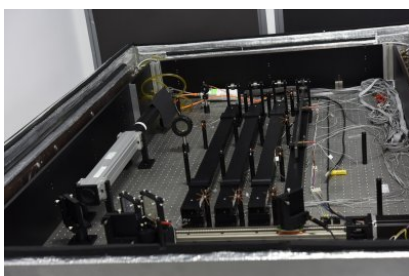
Automatyczny interferometr multispektralny do wzorcowania długich płytek wzorcowych
