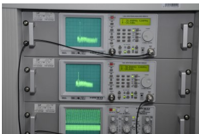
Fragment państwowego wzorca jednostki długości - syntezer częstotliwości optycznych (układ elektroniczny)
