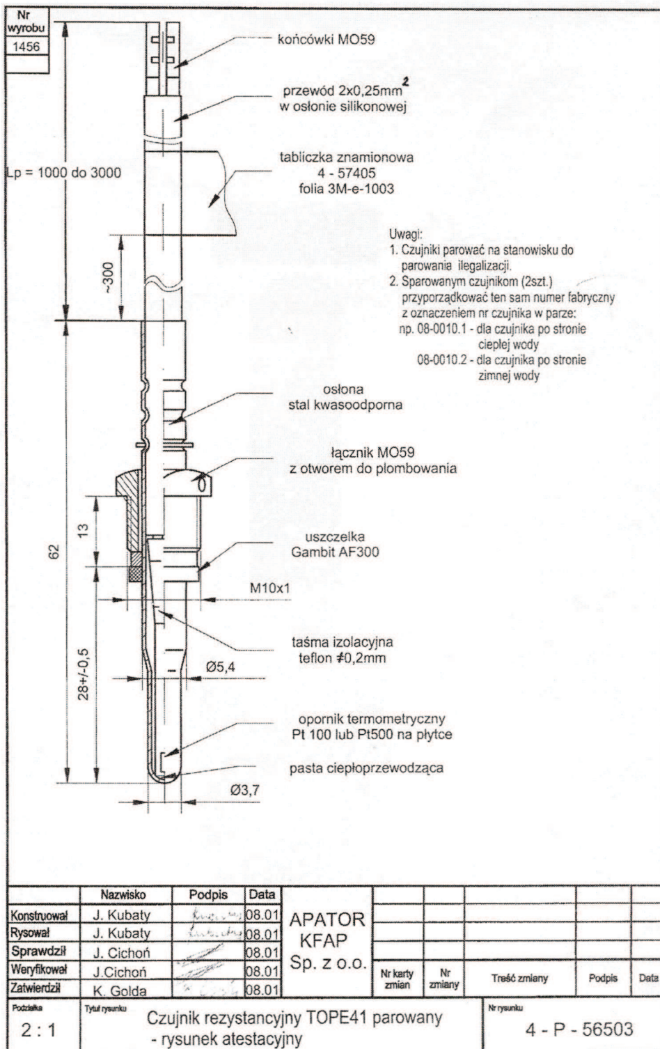
Rysunek 1. Czujnik rezystancyjny TOPE 41 parowany - rysunek atestacyjny.
